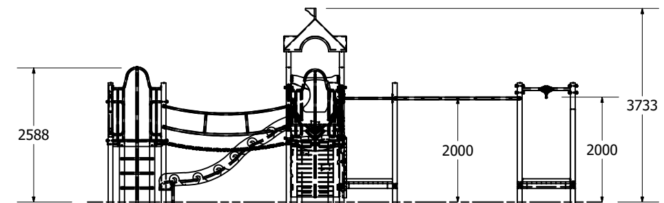
Right Elevation
