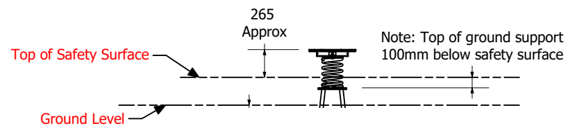
Right Elevation
